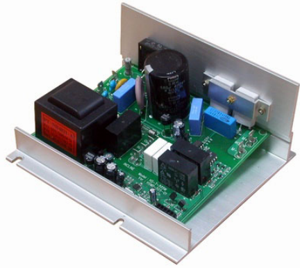
Tunturi와 Life-fitness에 OEM 공급하는 컨트롤러(PCB)
