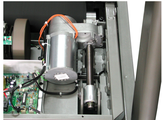
미국,대만,한국,중국특허의 전방 충격흡수 인크라인구조 (특허 NO.
