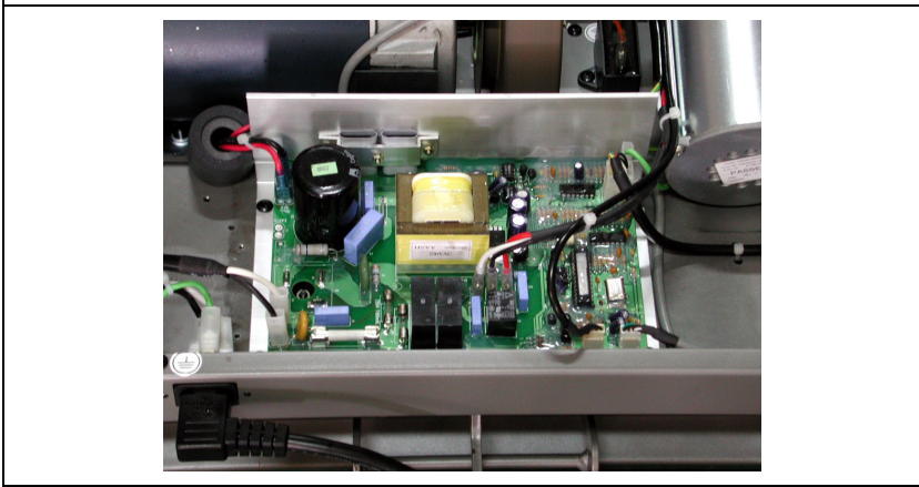
컨트롤러(PCB)
