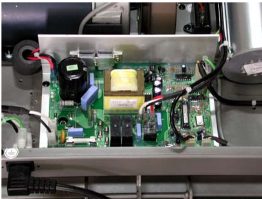
컨트롤러(PCB)
