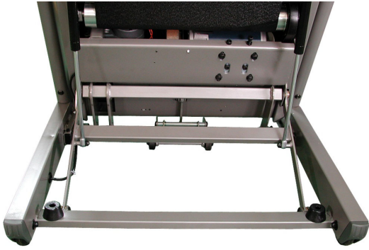
전후 4개의 이동바퀴
