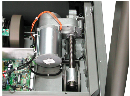
경사 조절용 모터(Incline Motor)
