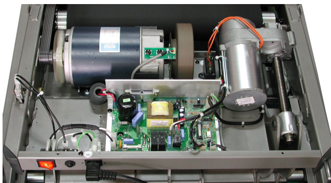
모터실 전경
