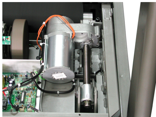
경사 조절용 모터(Incline Motor)
